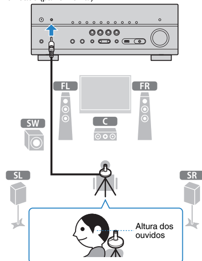
A unidade (painel frontal)
