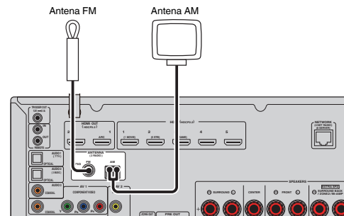
A unidade (painel traseiro)
