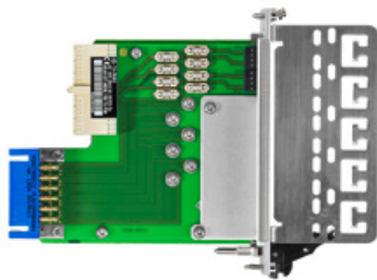
R&S®TS-PRIO3, rear I/O module for R&S®TS-PSM3
