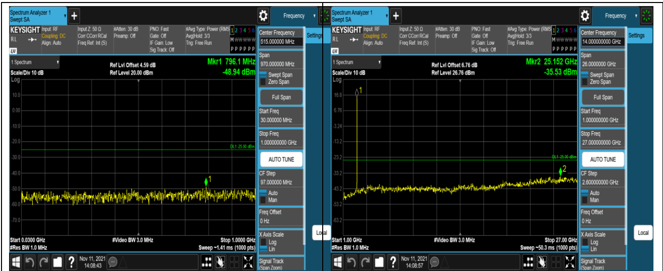
Band7-5MHz-QPSK-21100-1RB#0-Range1:30~100 0MHz
