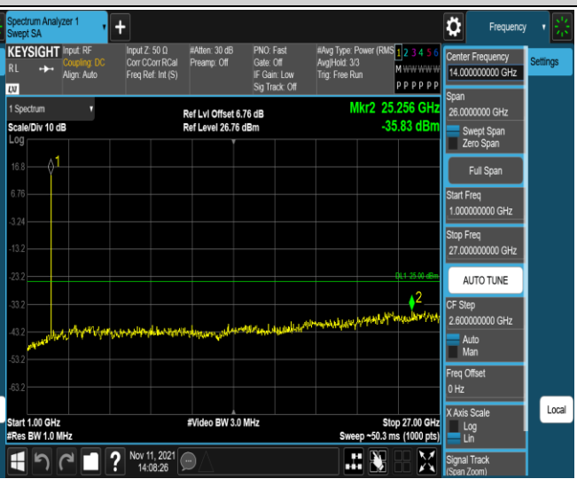
Band7-5MHz-QPSK-21425-1RB#0-Range2:1000~270 00MHz
