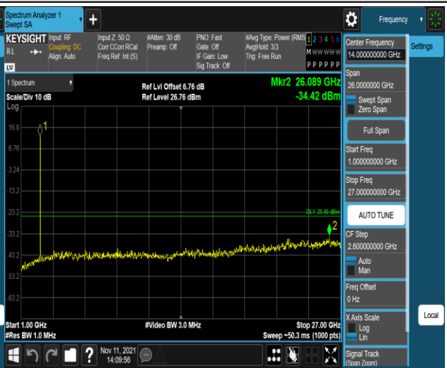
Band7-5MHz-QPSK-21425-1RB#0-Range2:1000~270 00MHz
