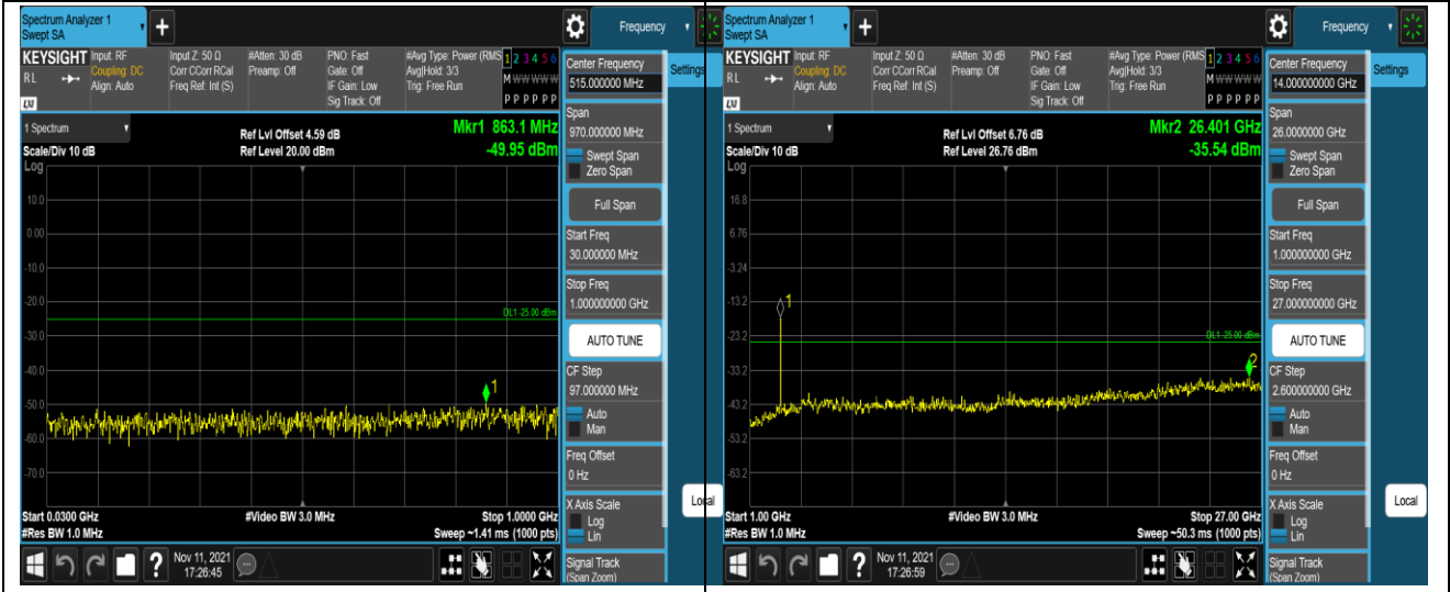
Band7-20MHz-QPSK-21100-1 RB#0-Range 1:30~1000MHz Band7-20MHz-QPSK-21100-1 RB#0-Range 2: 1000~27000MHz
