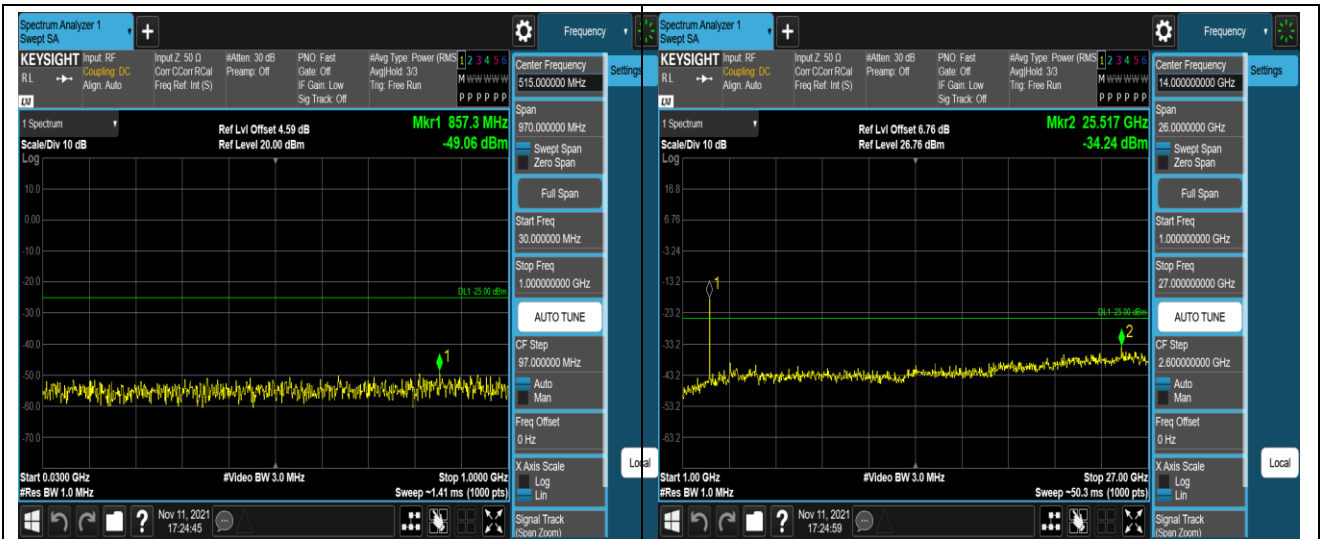
Band7-20MHz-QPSK-20850-1 RB#0-Range 1:30~1000MHz Band7-20MHz-QPSK-20850-1 RB#0-Range 2: 1000~27000MHz
