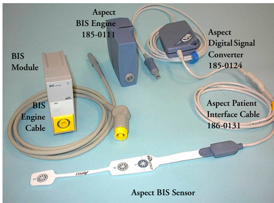
Figure 14 BIS Solution Components with BIS Engine and DSC
