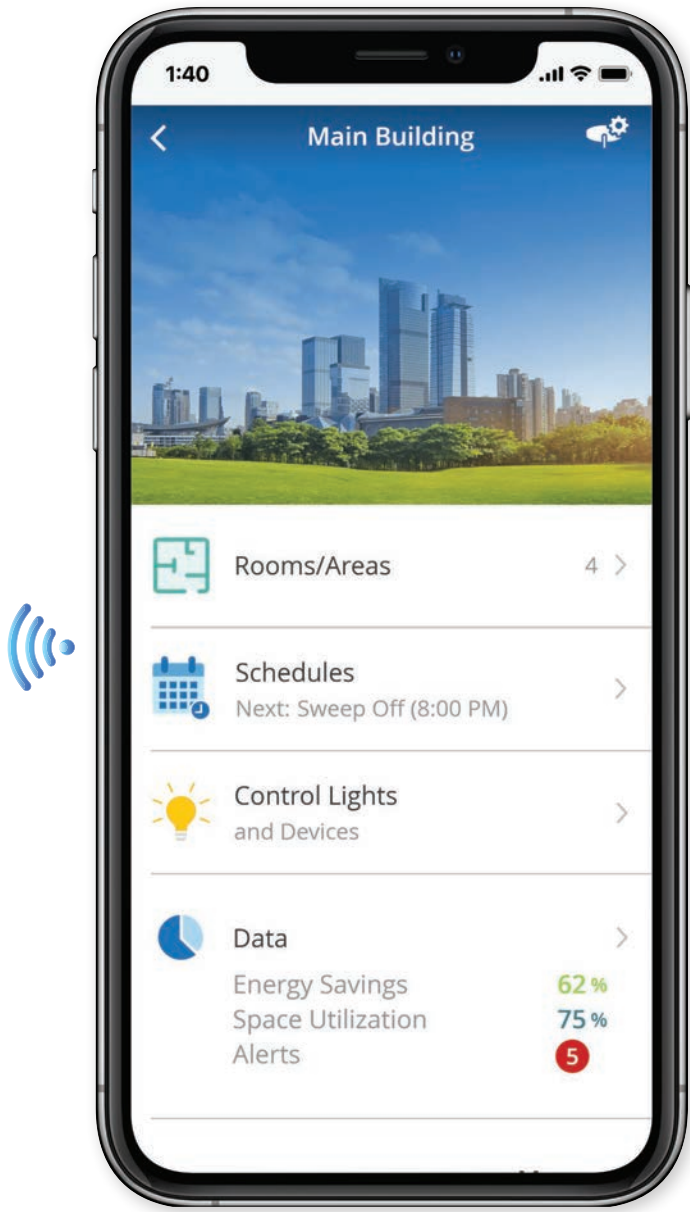
Vive software
