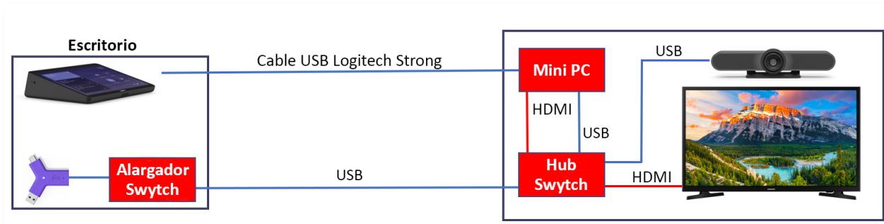
Figura 5: diagrama de instalación de la solución de Logitech para salas pequeñas, incluidos Logitech Tap, MeetUp y Swytch
