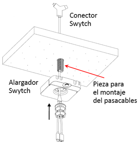
Figura 8: extensor Logitech Swytch, montaje de ojal bajo la mesa
