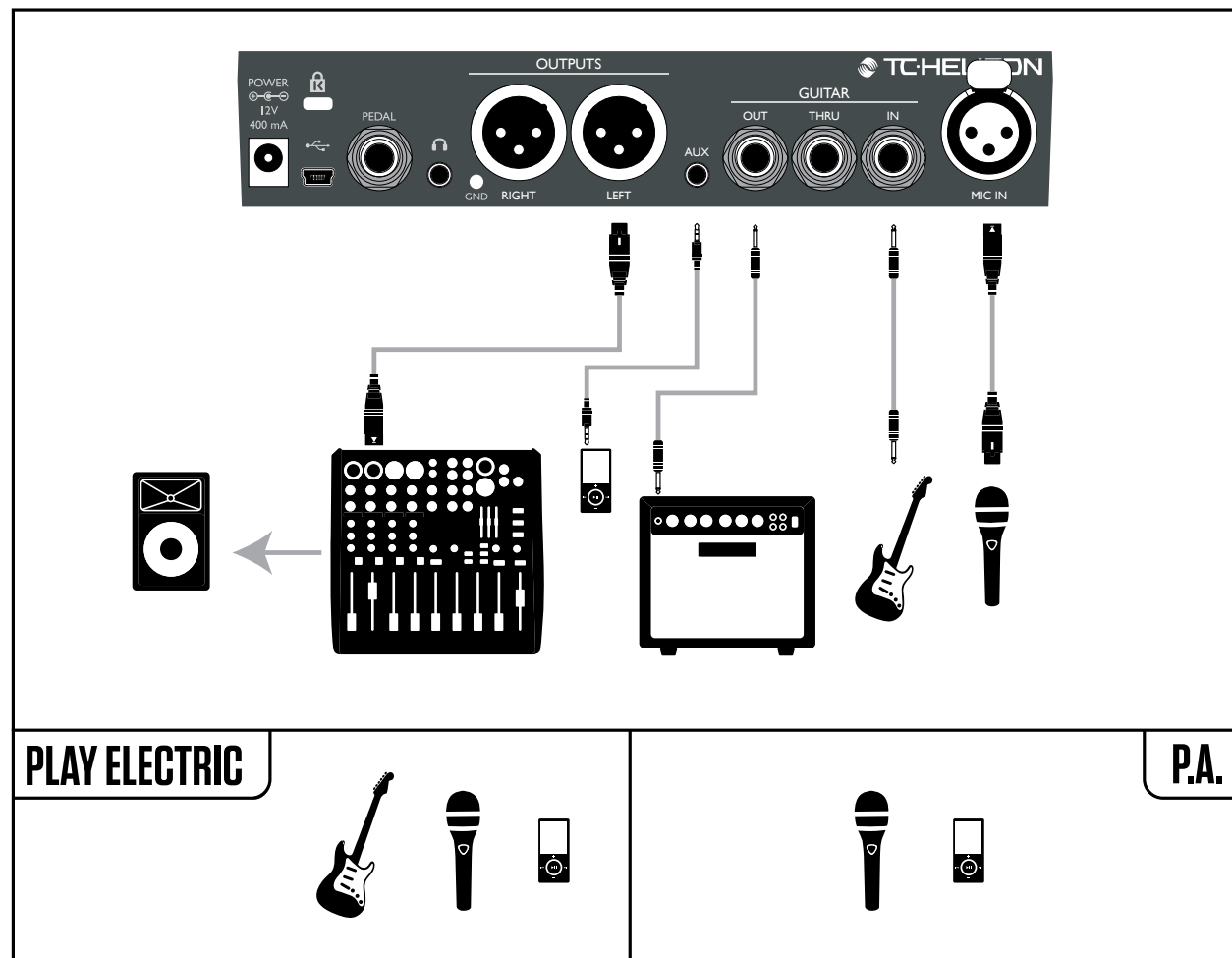
Ejemplo de configuración: Voces en mono y amplificador de guitarra
