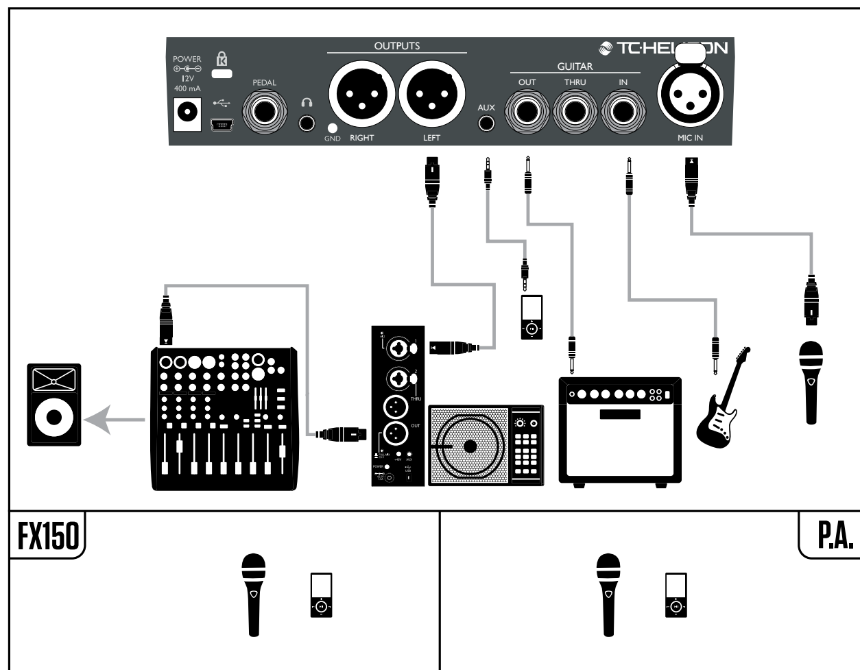
Ejemplo de configuración: Voces en mono a través de un FX150 y un amplificador de guitarra
