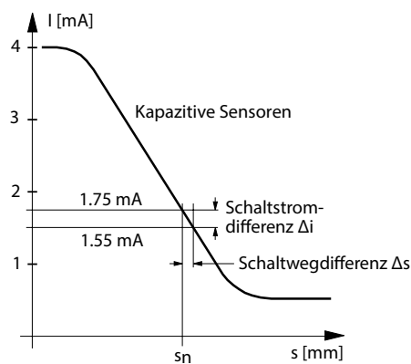
Abb. 1: NAMUR-Kennlinie der kapazitiven Sensoren gemäß EN 60947-5-6
