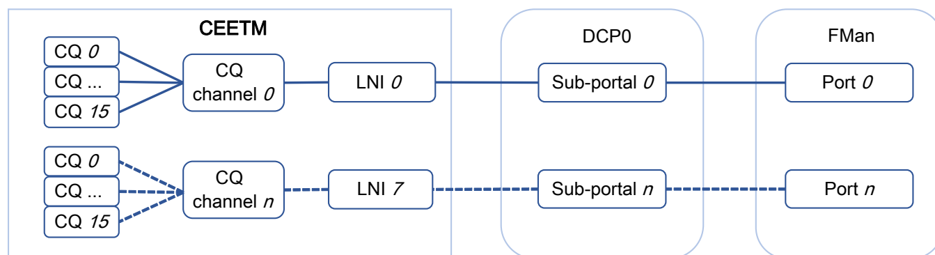
Figure 89. CEETM block
