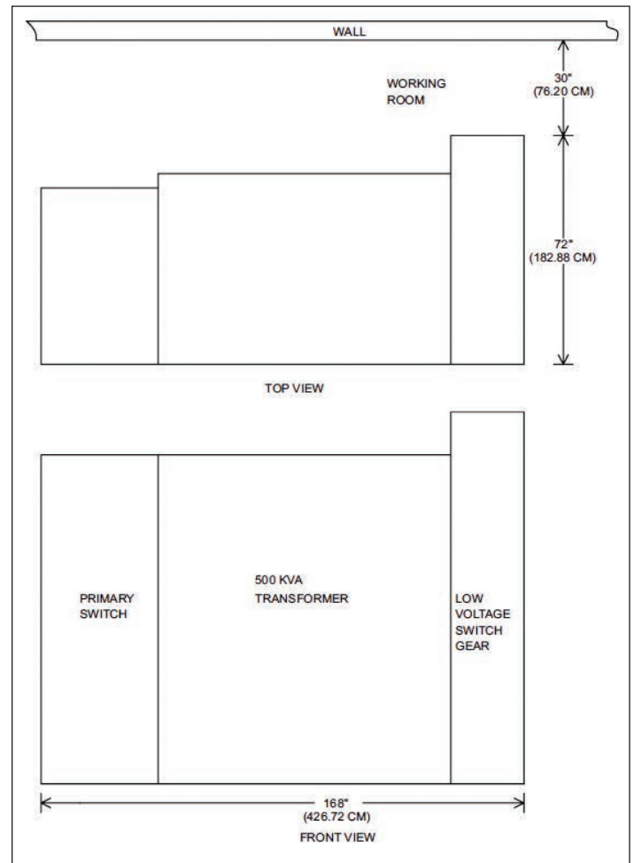
Figure 7. Conventional SUS
