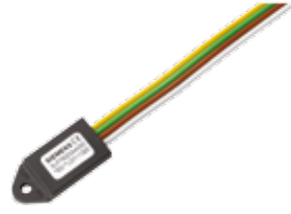
Módulo Inicialización
