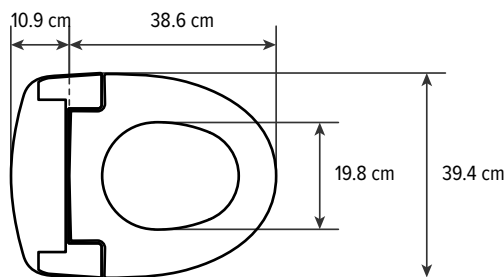
Vista Superior Redonda
