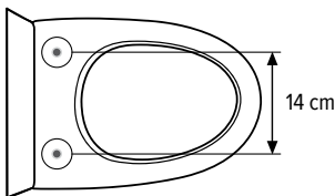
Distancia Entre los Orificios de Montaje
