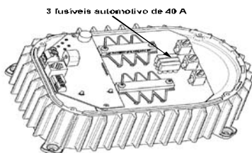
Fig. 8 Localização dos fusíveis
