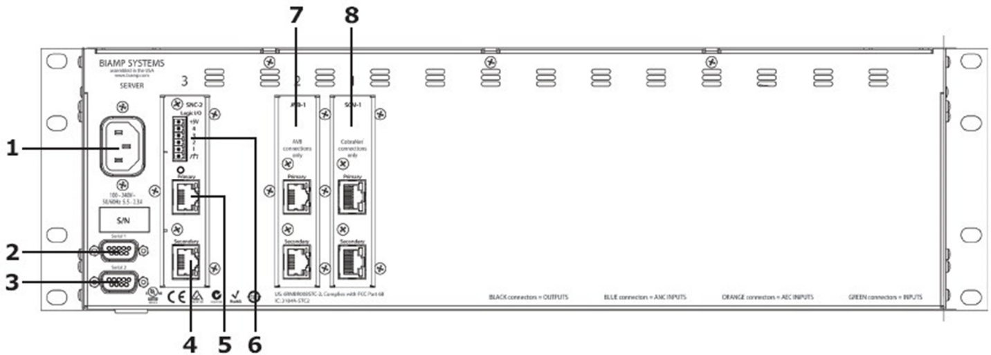
Tesira SERVER
