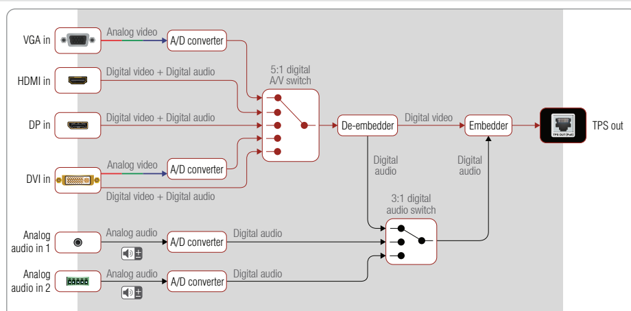
Port Diagram - UMX-TPS-TX140
