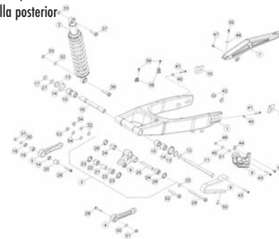
TAV.33 Forcellone posteriore - Rear fork - Fourche arrière - Hinterradschwinge - Horquilla posterior
