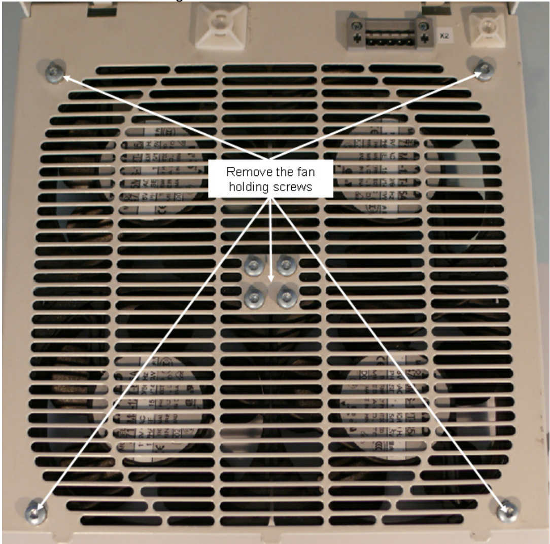
Fan holding screws
