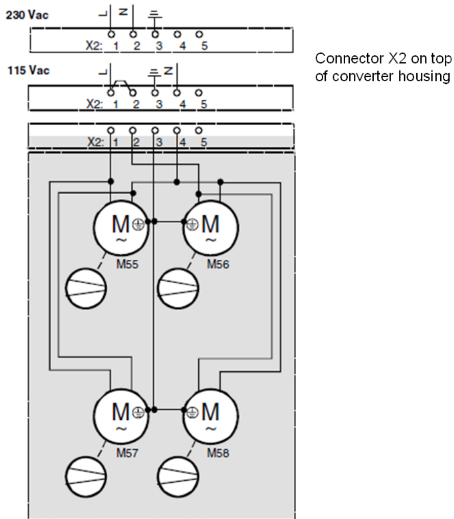
Fan configuration D3
