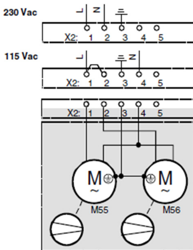
Fan configuration D1 to D3
