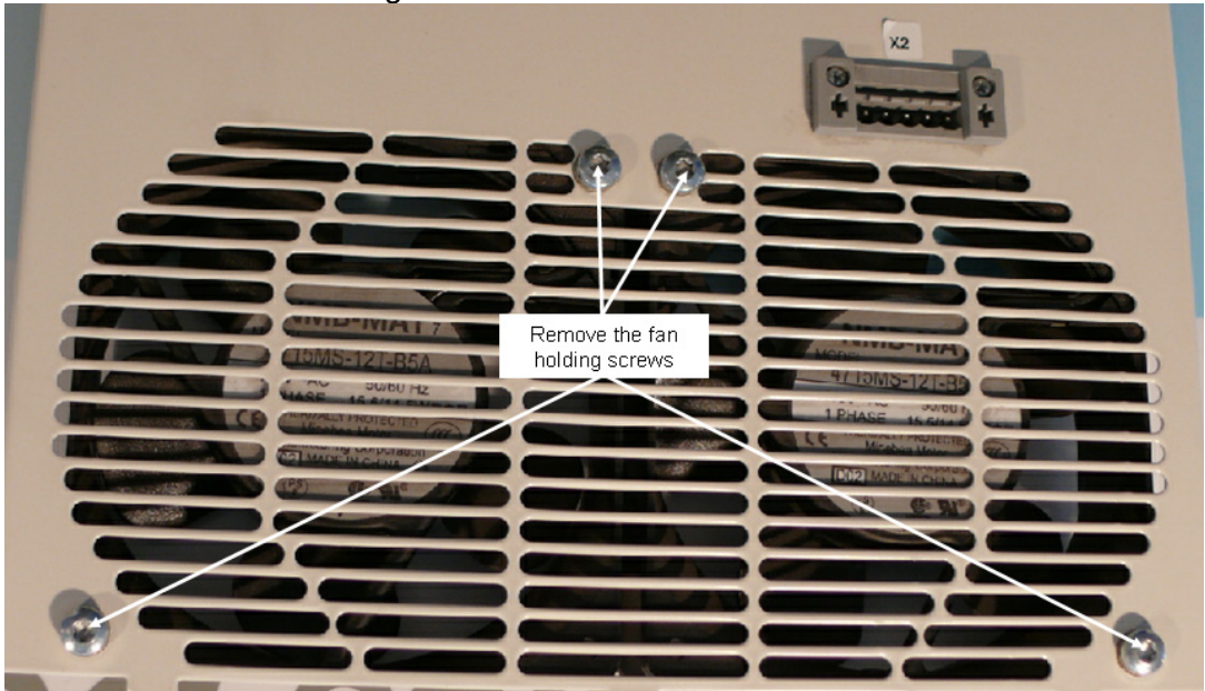
Fan holding screws
