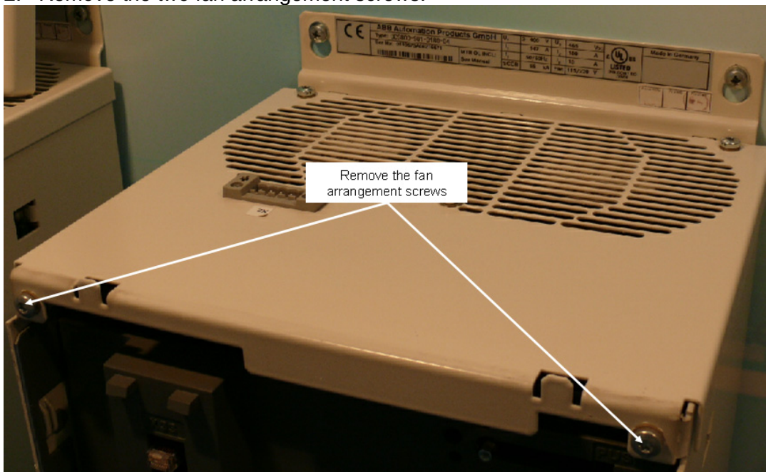
Fan arrangement
