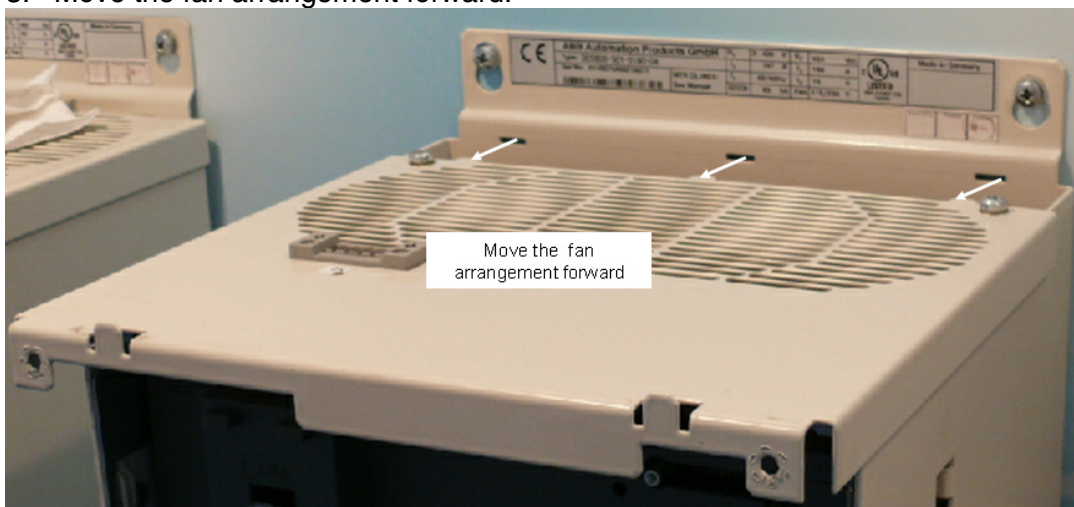
Move fan arrangement
