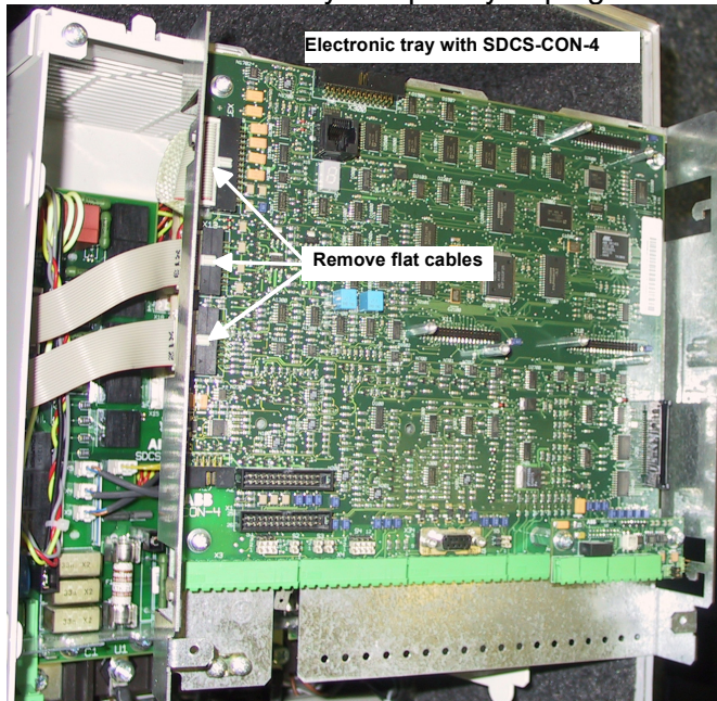
Unhinge electronic tray
