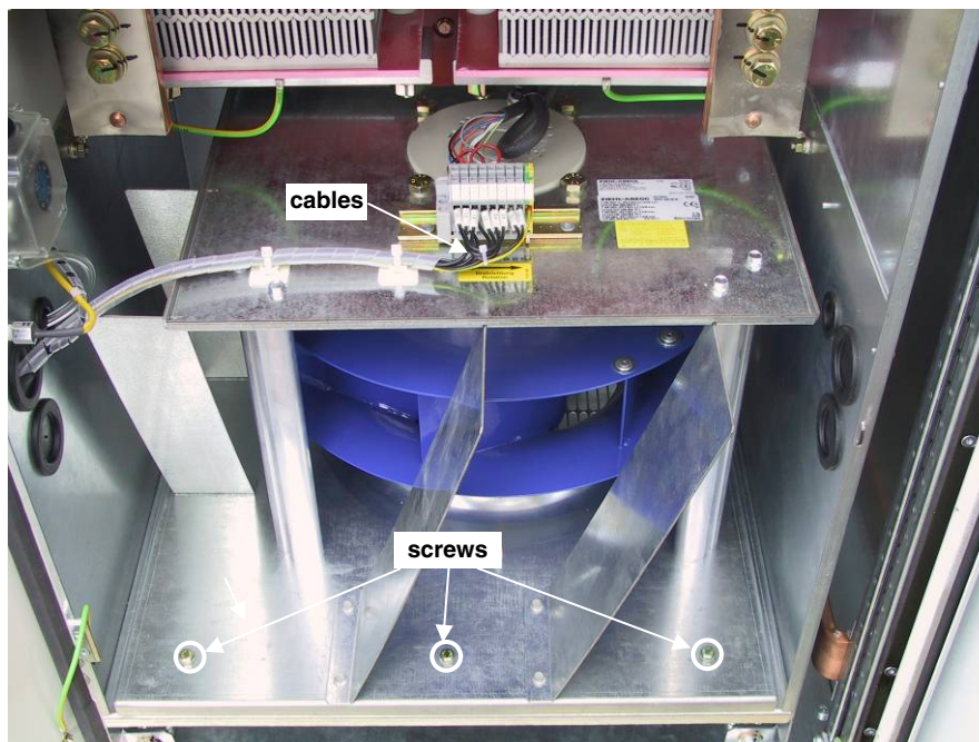
Converter fan in frame D7
