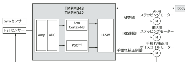
システムブロック図(カメラレンズ)
