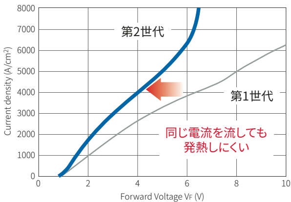
電流サージ耐量 I FSM が 70% 改善
