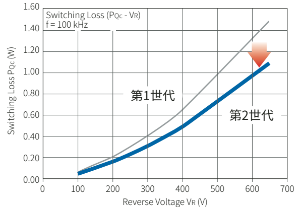
スイッチング損失を 30% 低減 (650V、10A 品の例)
