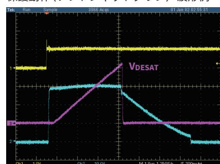
保護動作(ソフトシャットダウン) 波形例
