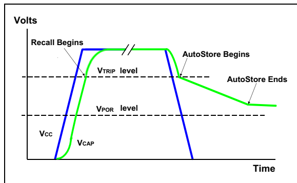
FIGURE 3: AUTOSTORE VOLTAGES
