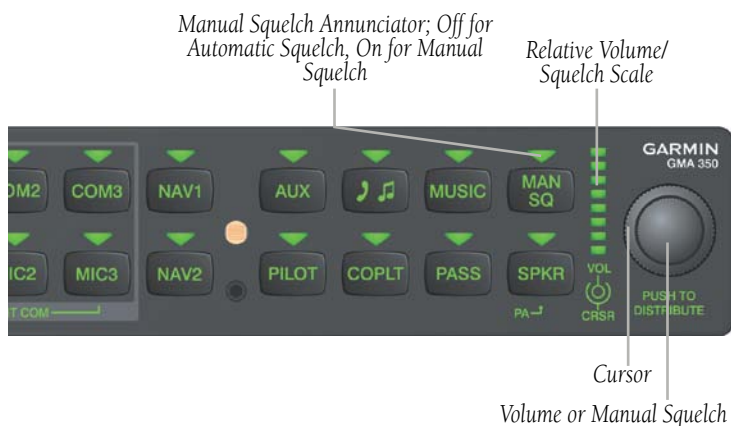
Volume/Squelch Control
