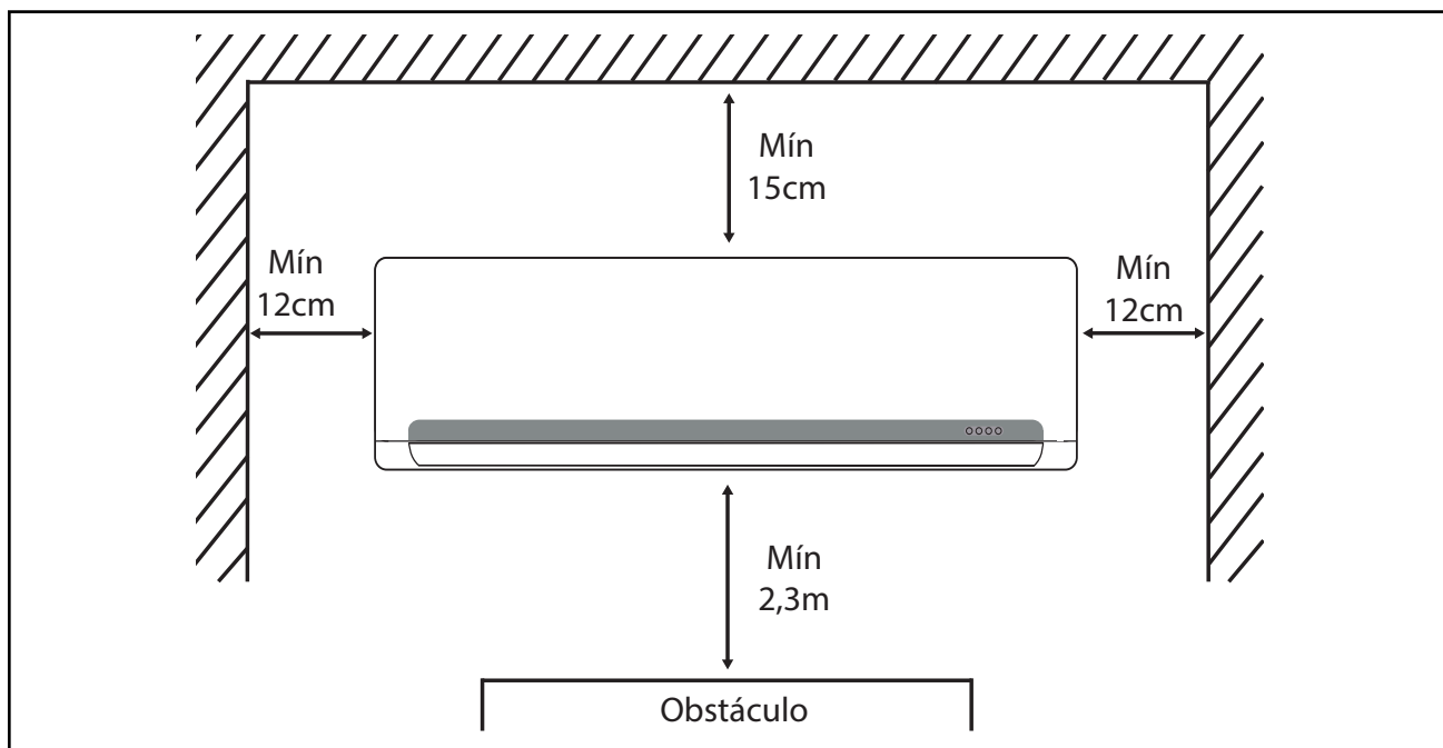
FIG. 13 - ESPAÇAMENTOS MÍNIMOS RECOMENDADOS
