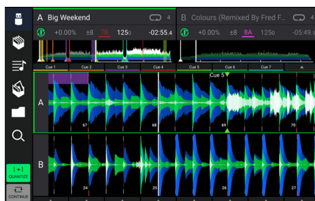
Visualizzazione delle onde a a strato doppio
