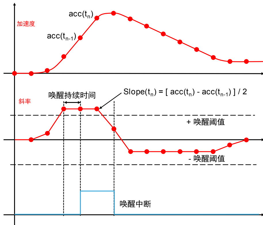
图 13. 唤醒中断（利用斜率滤波器）
