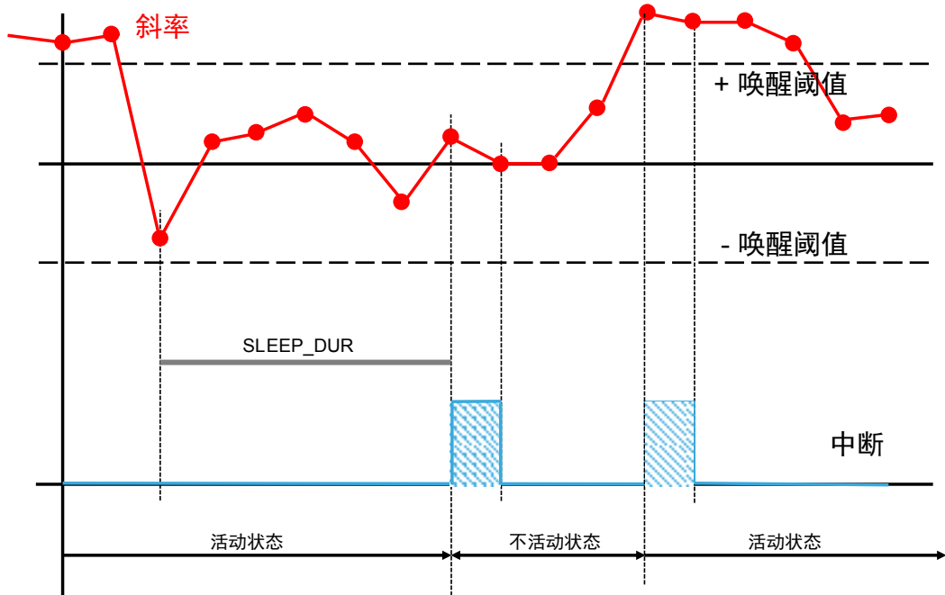
图 18. 活动/不活动识别（利用斜率滤波器）
