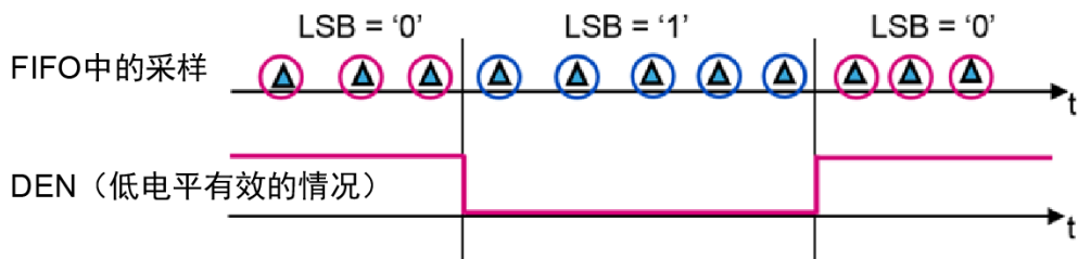
图 7. 电平感应触发模式，DEN 低电平有效
