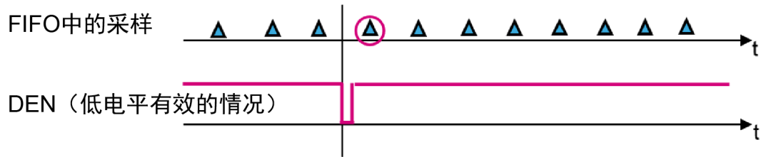
图 9. 电平感应锁存模式，DEN 低电平有效
