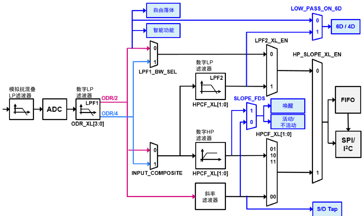
图 2. 加速度计滤波链
