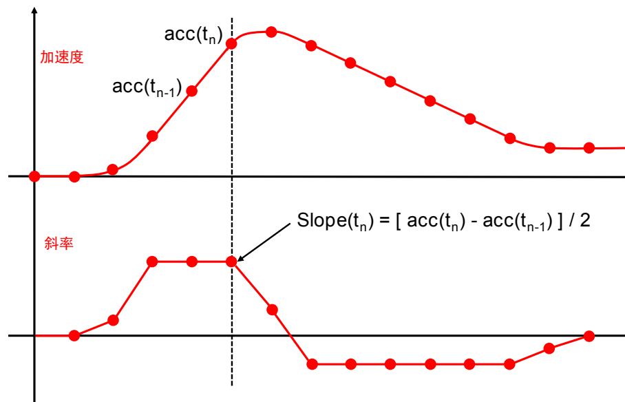
图 3. 加速度计斜率滤波器
