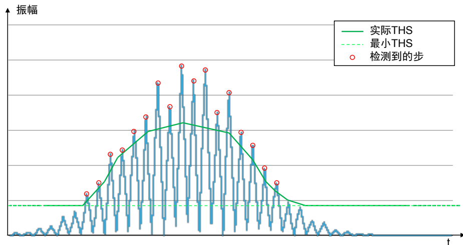
图 20. 计步器最小阈值
