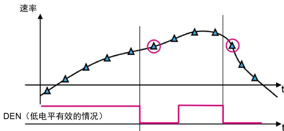
图 6. 边沿感应触发模式, DEN 低电平有效
