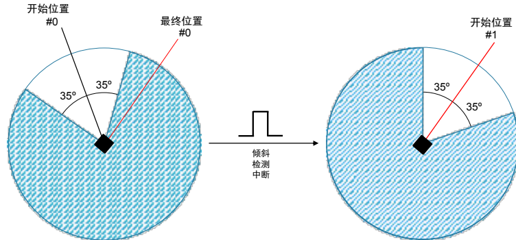
图 21. 倾斜度检测
