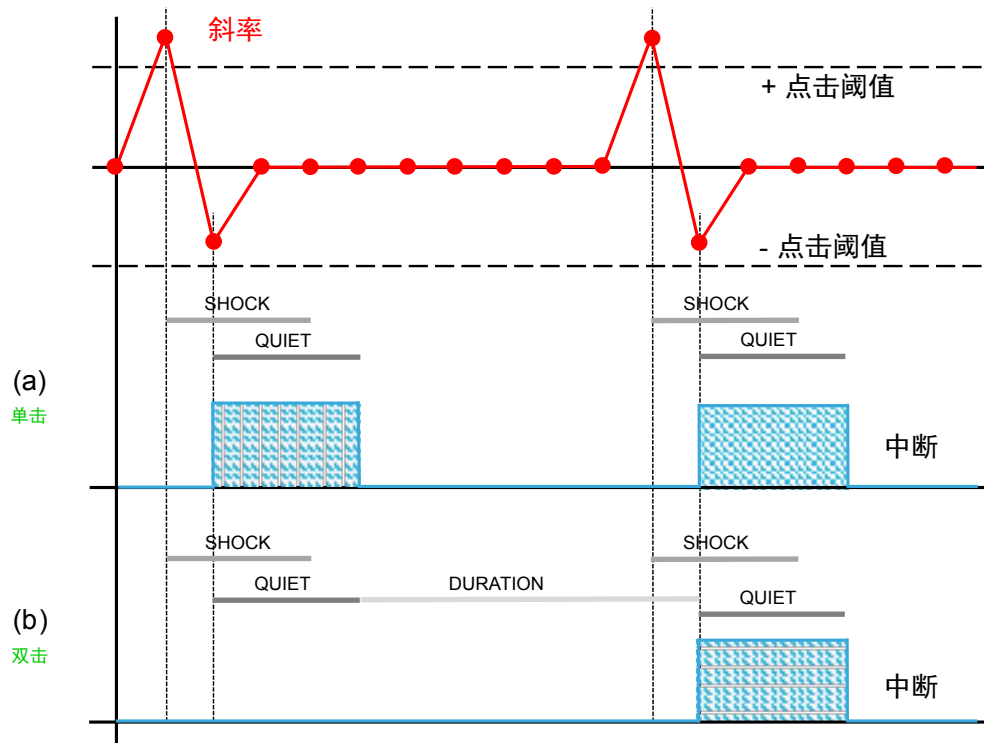
图 17. 单击和双击识别（LIR 位 = 0）
