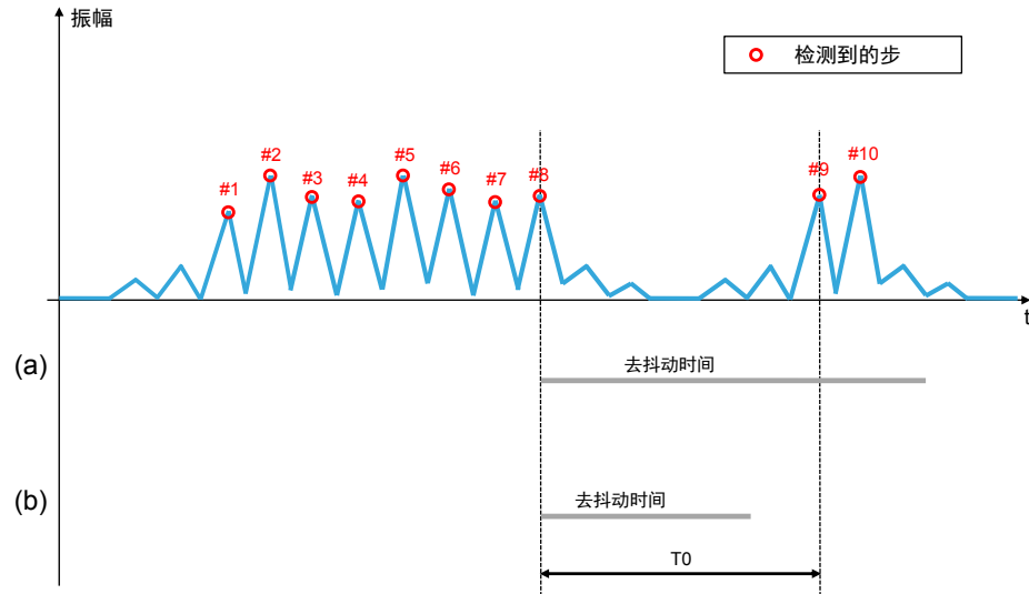
图 19. 计步器去抖动
