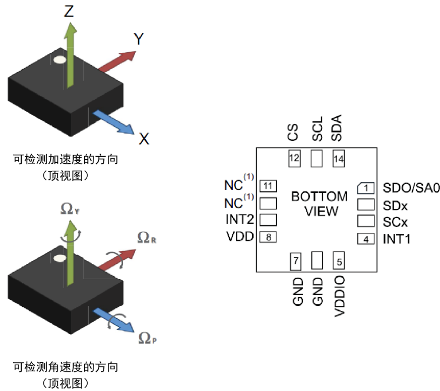
图 1. 引脚连接
