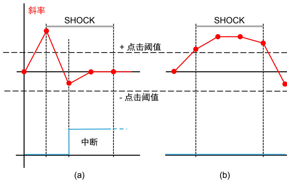
图 15. 单击事件识别
