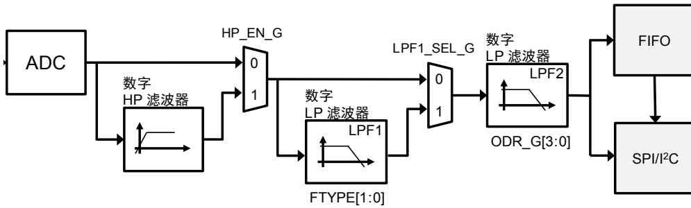
图 4. 陀螺仪数字链
