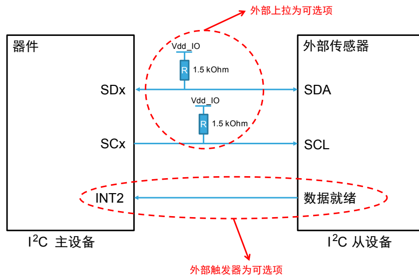
图 22. 模式 2 下外部传感器连接
