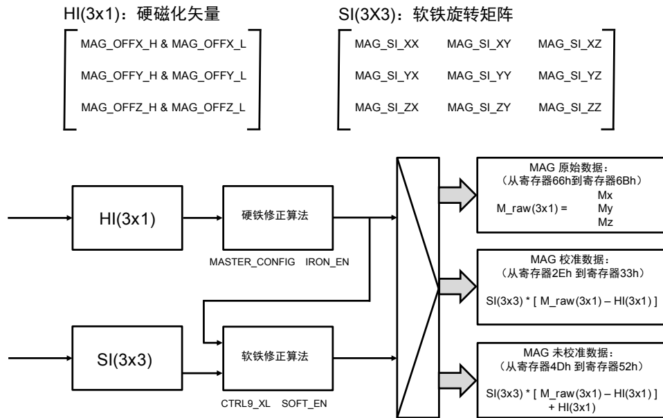
图 27. 硬磁/软磁校准框图
