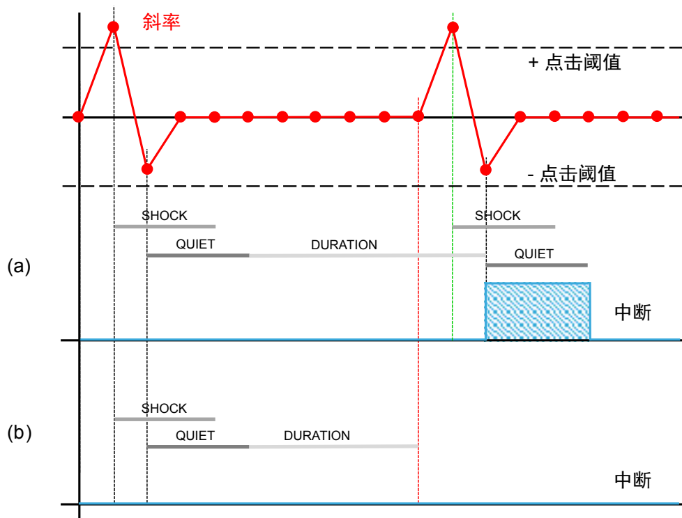
图 16. 双击事件识别 ( LIR 位 = 0 )
