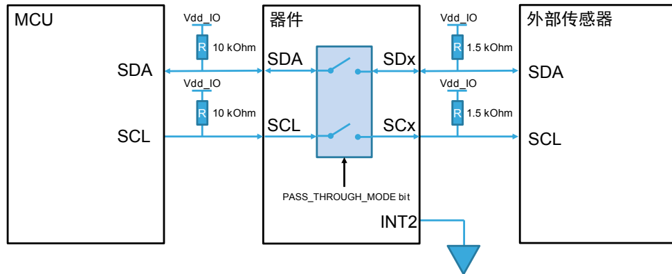
图 24. 直连功能
