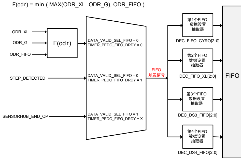
图 32. FIFO 触发信号选择
