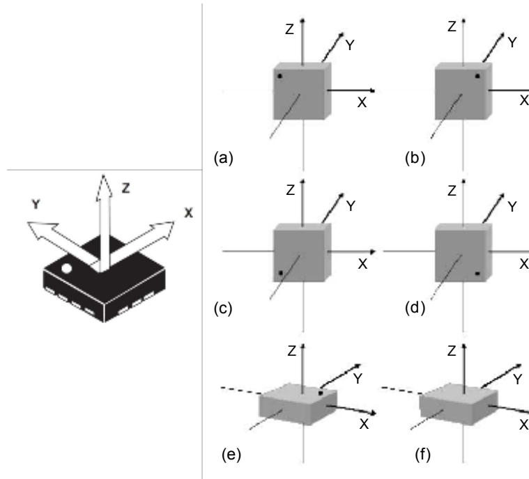
图 14. 6D 识别方向
