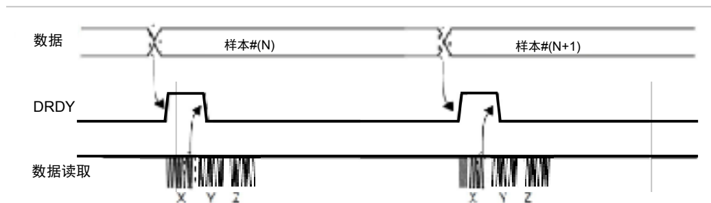
图 5. 数据准备就绪信号
