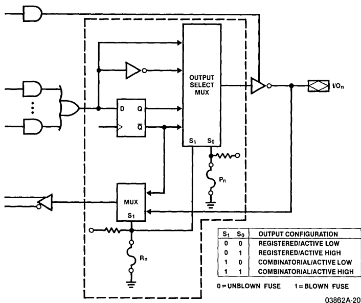
AmpPAL22V10 Output Logic Macrocell
