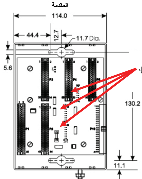
الشكل 2. أبعاد مبيت ControlWave Micro الأساسي رباعي الفتحات (بالمليمترات)
