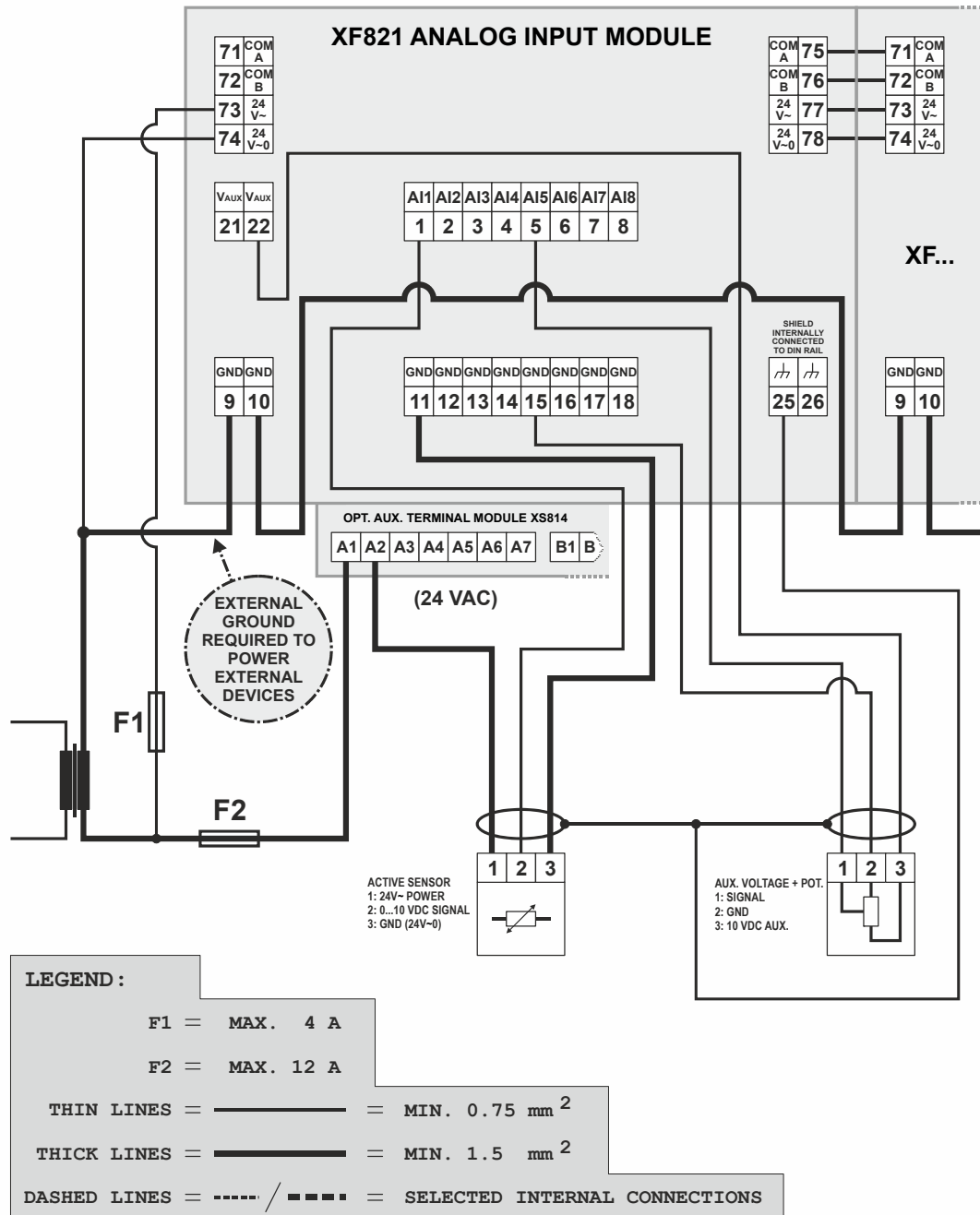
Fig. 33. Analog input module, wiring example 1
