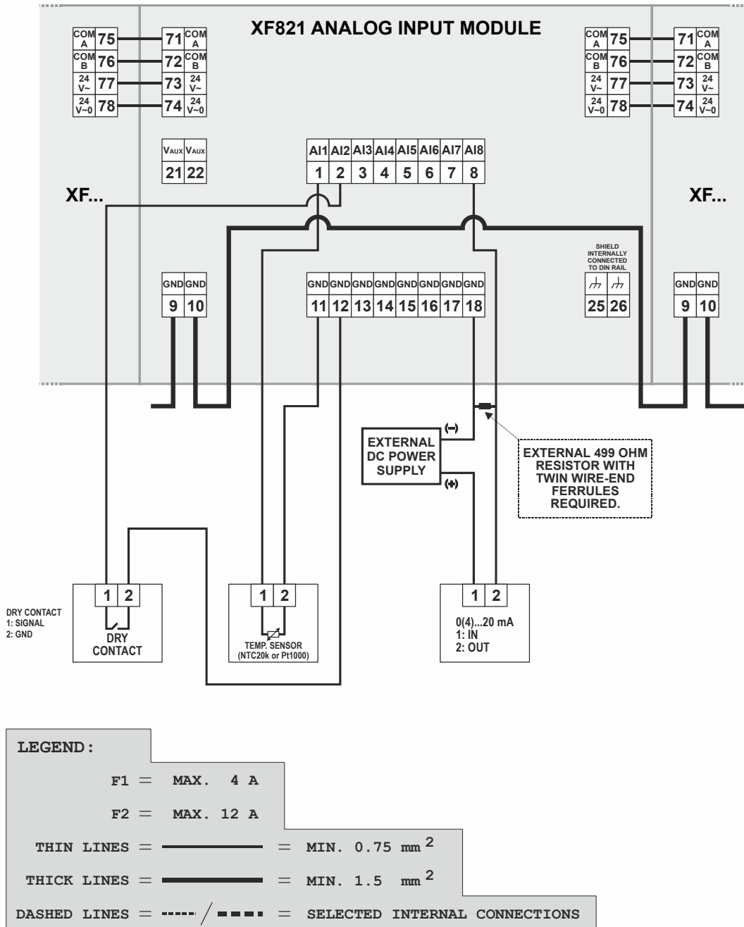
Fig. 34. Analog input module, wiring example 2
