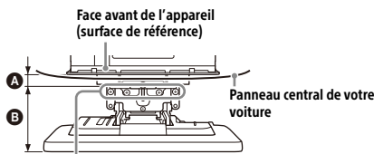
Positions des trous de vis (pour fixer l'écran et l'appareil)
