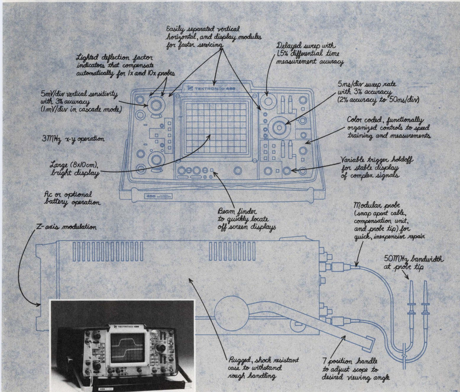
TEKTRONIX 455 — $1695
