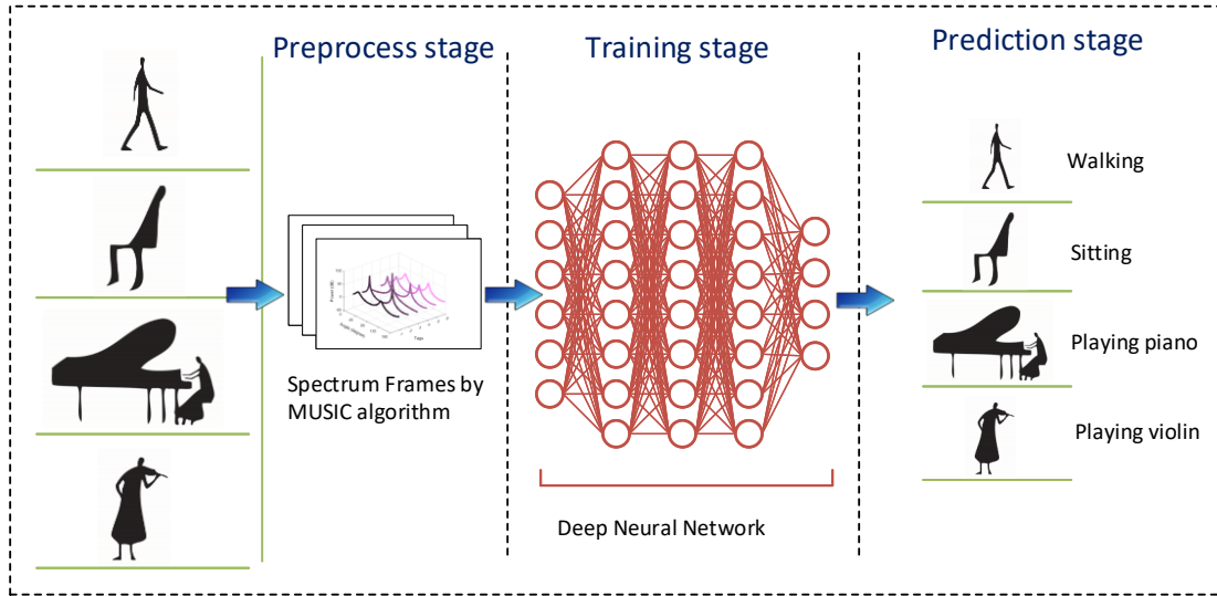
Fig. 5. TagFree framework
