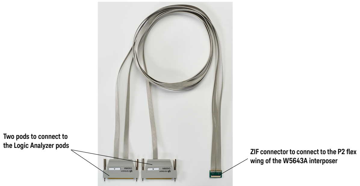
Figure 3 U4208A 61-pin ZIF probe cable
