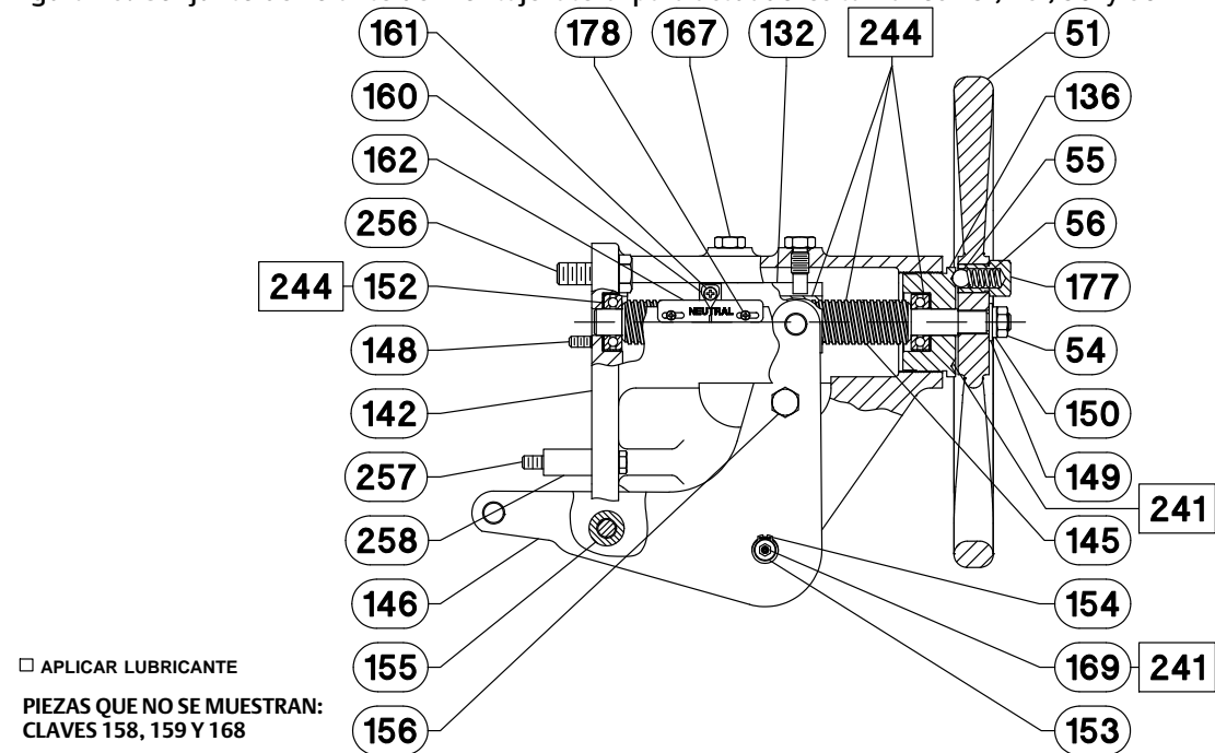
Figura 16. Conjunto de volante de montaje lateral para actuadores tamaños 45i, 46i, 50i y 60i
