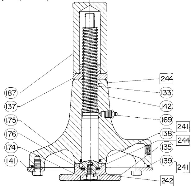
Figura 19. Tope de carrera ascendente ajustable montado en la caja para actuadores tamaños 70/70i y 87 (estilo 1)
