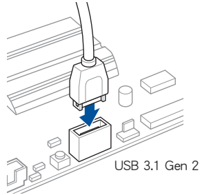
安装 USB 3.1 Gen 2 前面板连接端口
