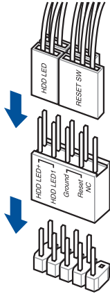
安装华硕 Q-Connector
