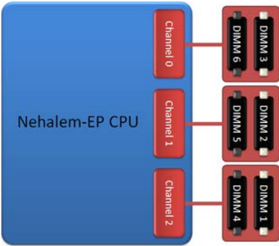
Configuración de ranura DIMM para un solo procesador o un segundo procesador en la tarjeta vertical.
