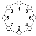
8-Lug Nuts
