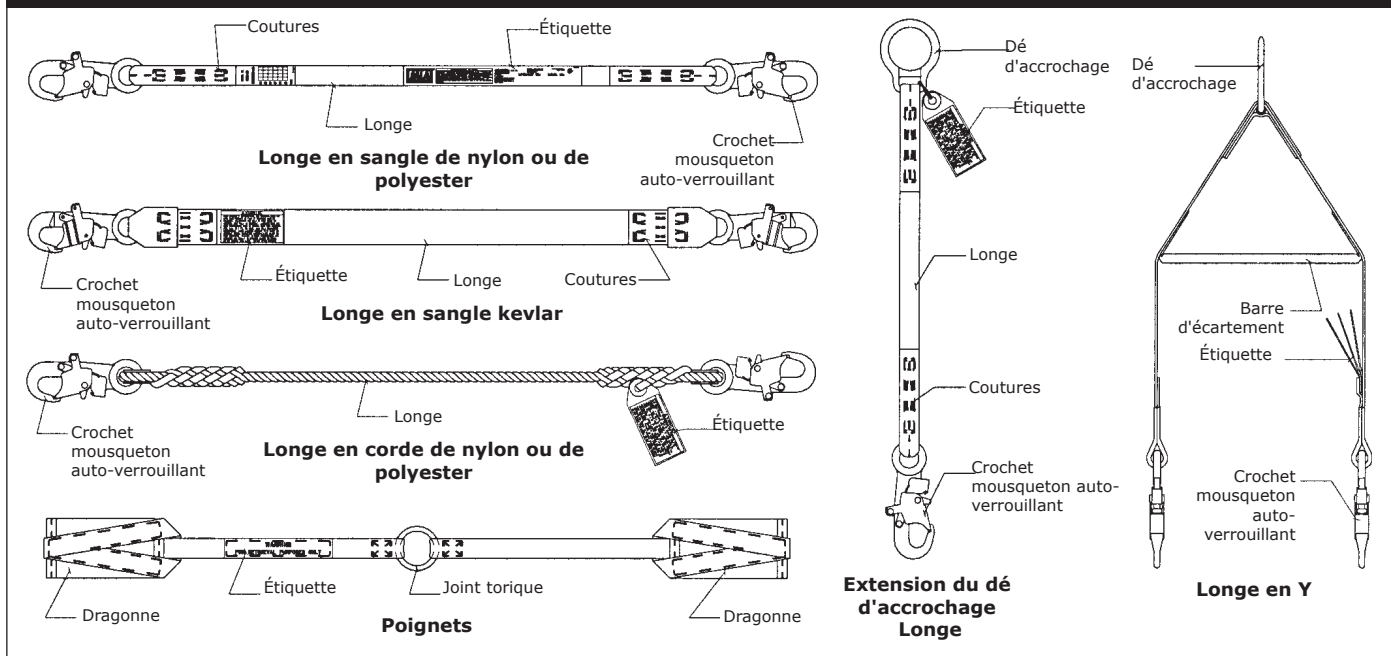
Figure 1 - Longes en sangle et en corde
