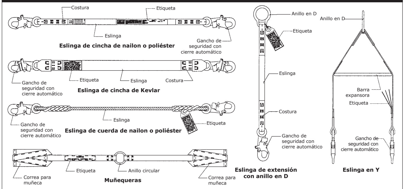
Figura 1 - Eslingas de cincha y de cuerda
