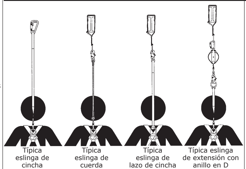
Figura 5 - Anclaje
