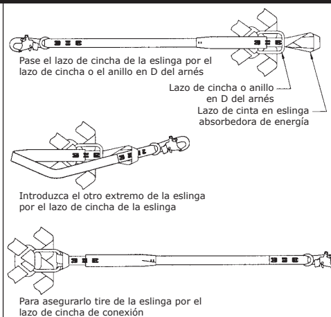
Figura 7 - Conexión del lazo de cincha
