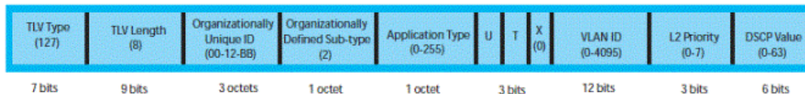
Figure 24. LLDP-MED Policies TLV
