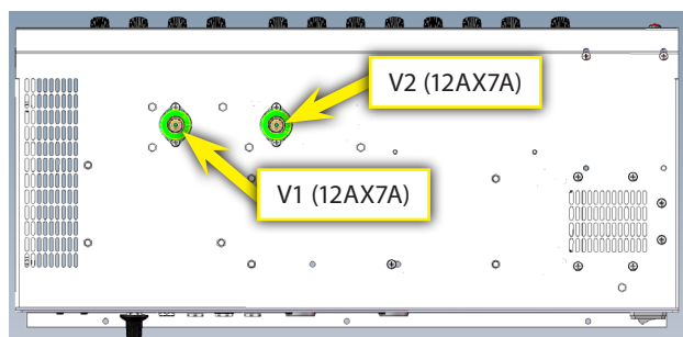
(šasi zespodu)
