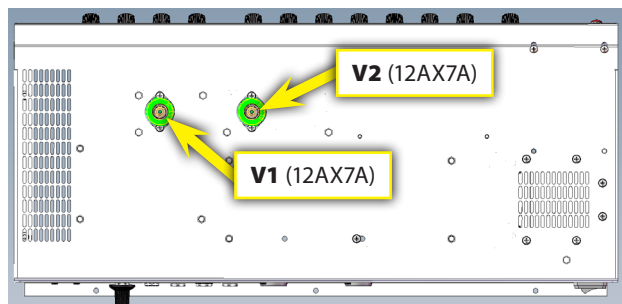
(Chassis, Unterseite)
