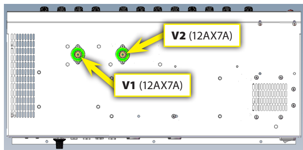
(机箱, 仰视图)
