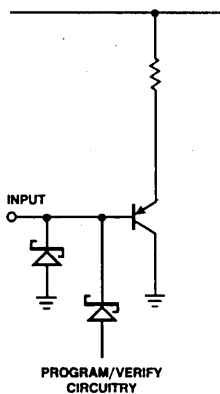
Input Circuitry
