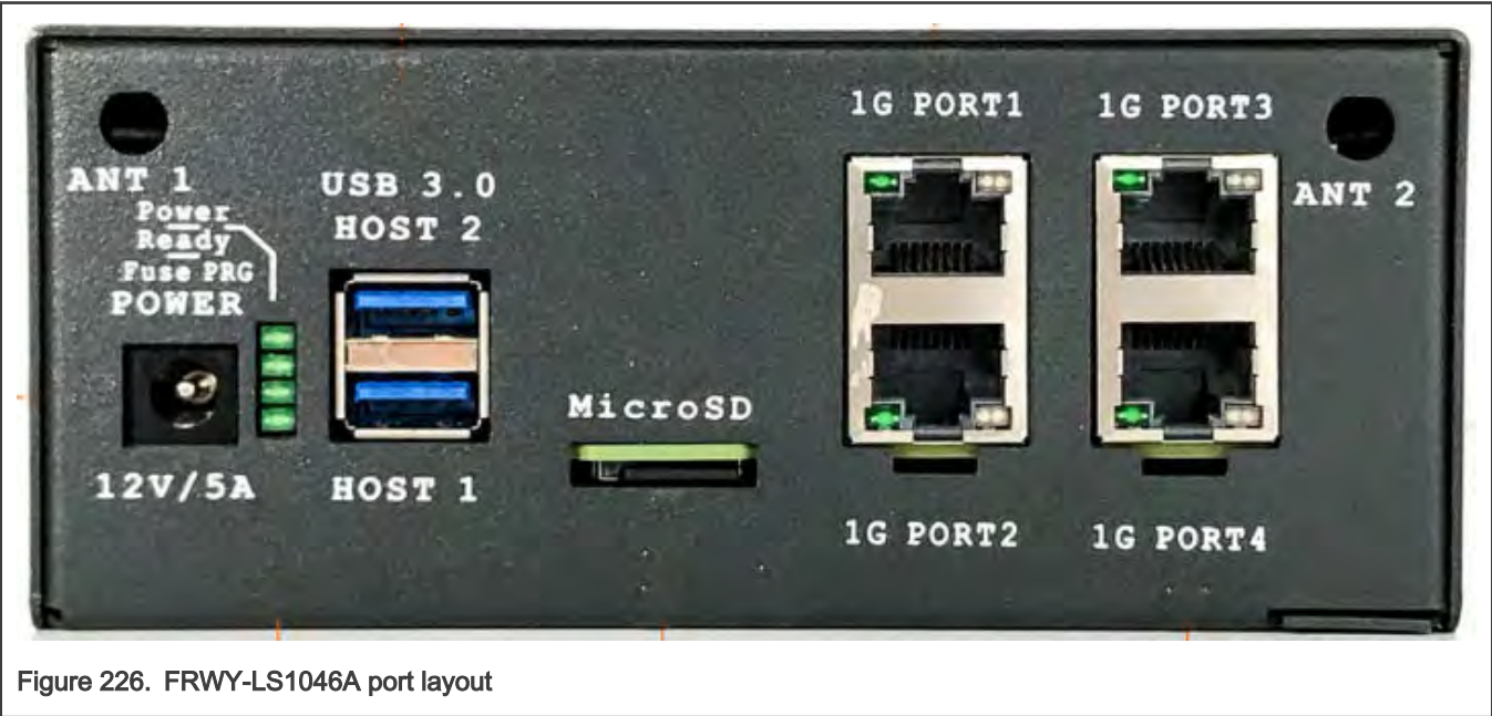
FRWY-LS1046A port layout
