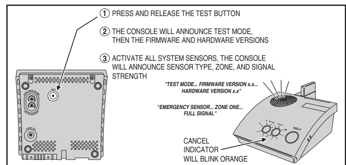
Test/Learn Mode
