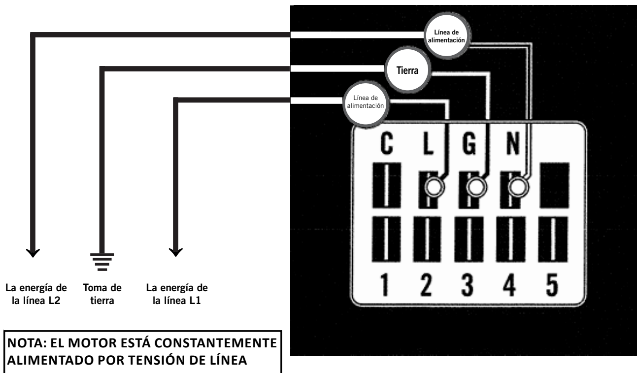
FIGURA 11 Conexiones del motor
