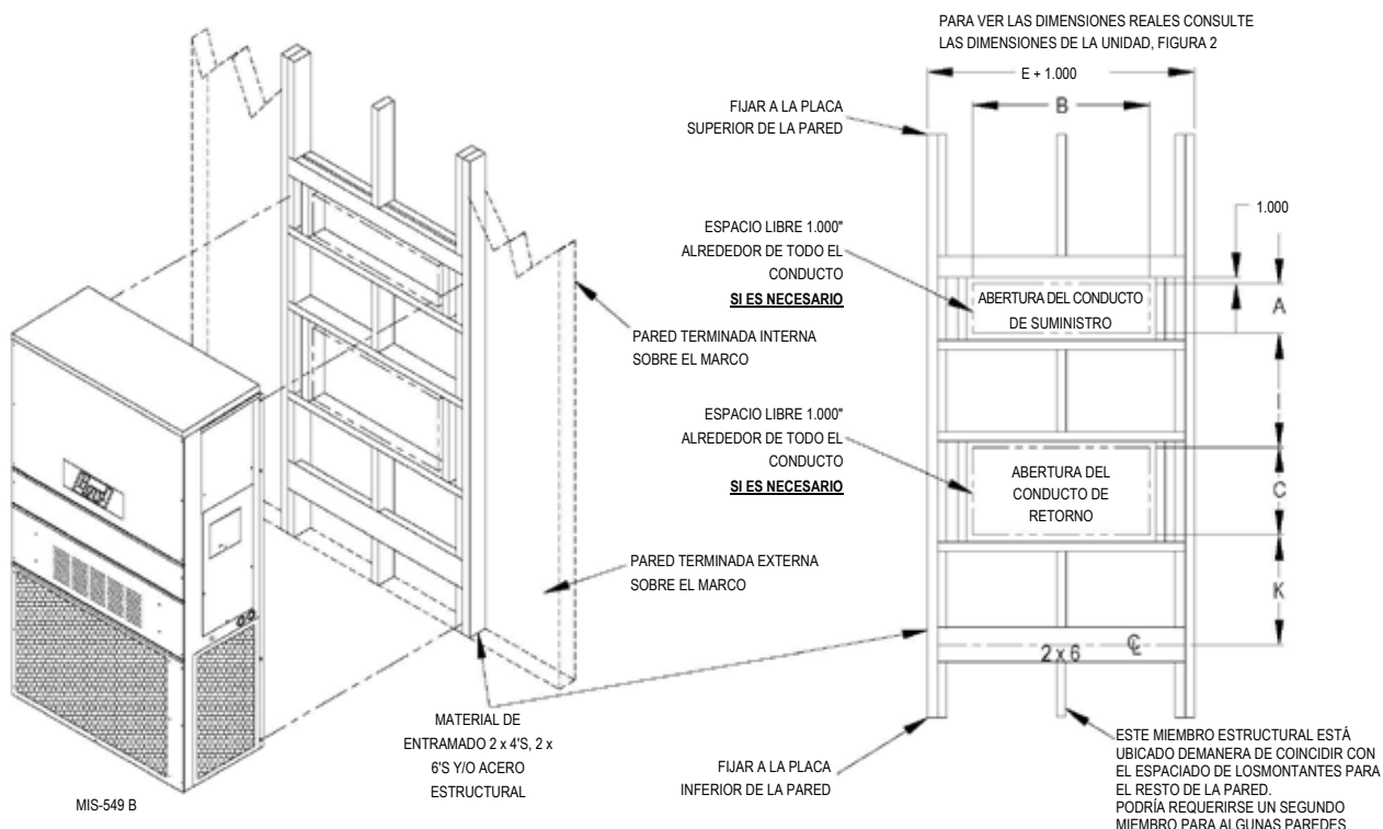
FIGURA 6 Instrucciones para montaje en la pared
