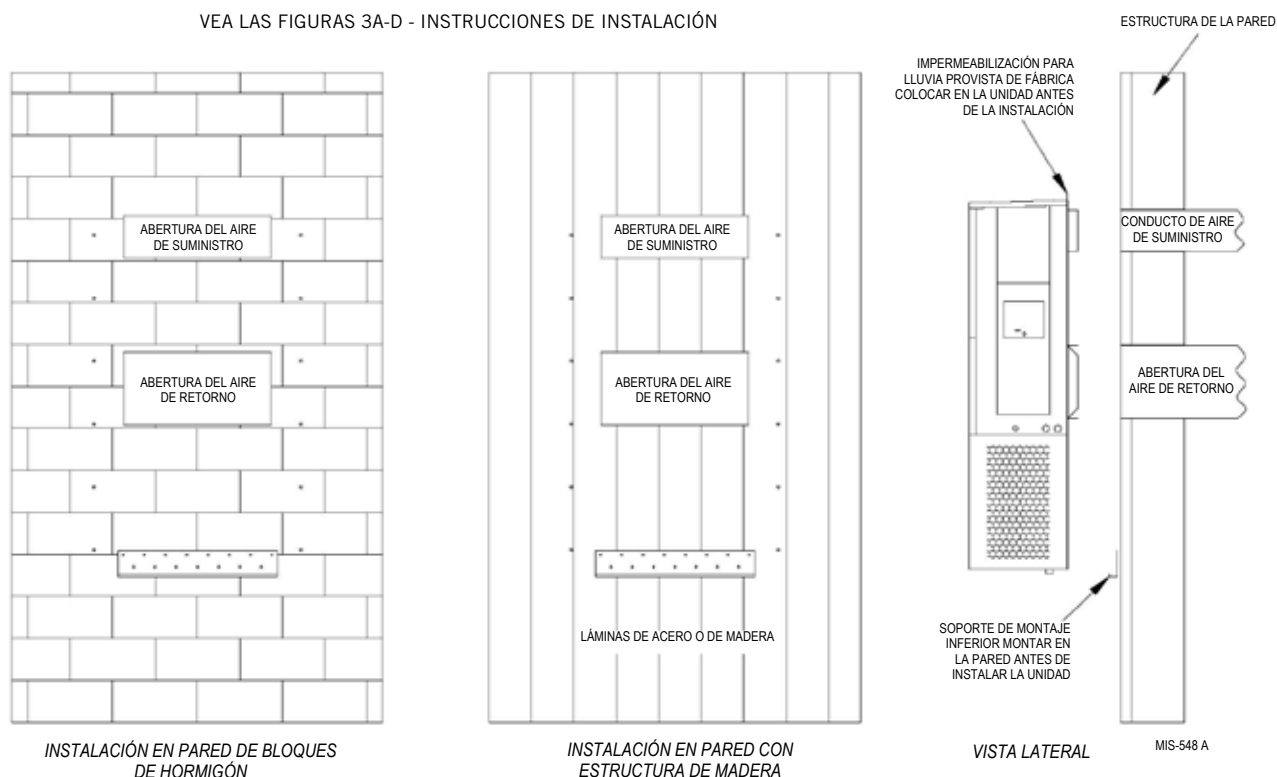
FIGURA 6 Instrucciones para montaje en la pared
