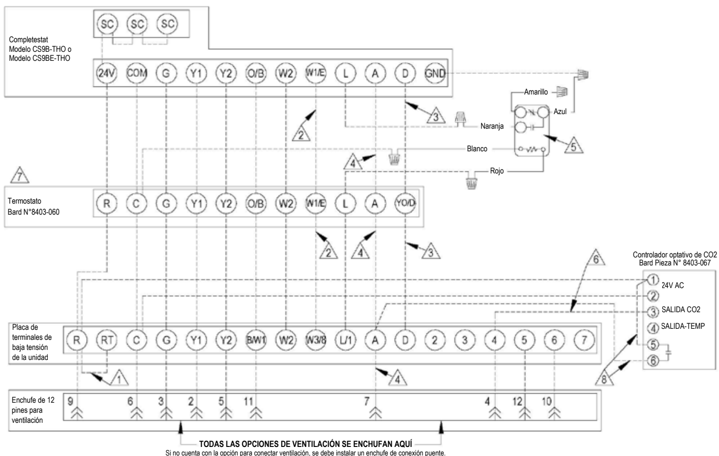
FIGURA 8 Conexiones para termostatos programables
