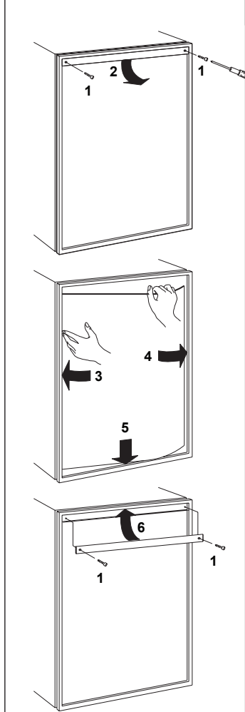
FIG 28 - DOOR PANEL
