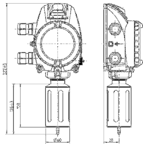
Fig. 30 Dimensions CalGard
