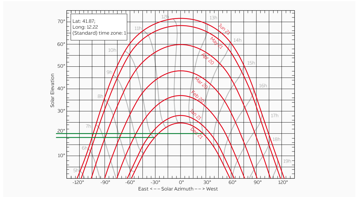
Figure 88 sun path in latitude 41.871730 and longitude 12.217600
