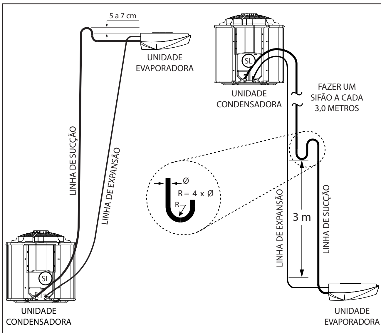
FIG. 23 - INSTALAÇÃO LINHAS DE INTERLIGAÇÃO
