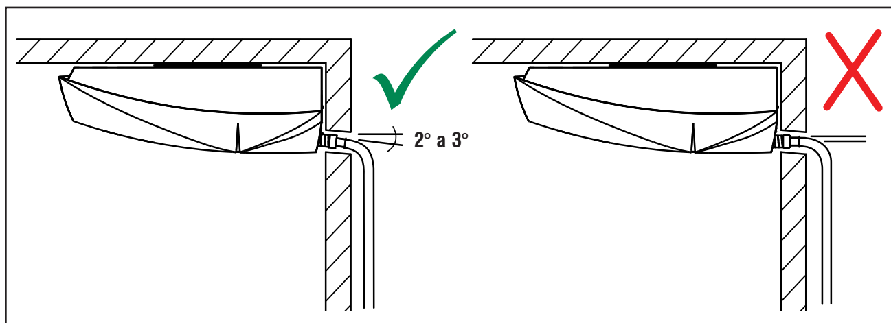
FIG. 21 - INCLINAÇÃO DRENAGEM
