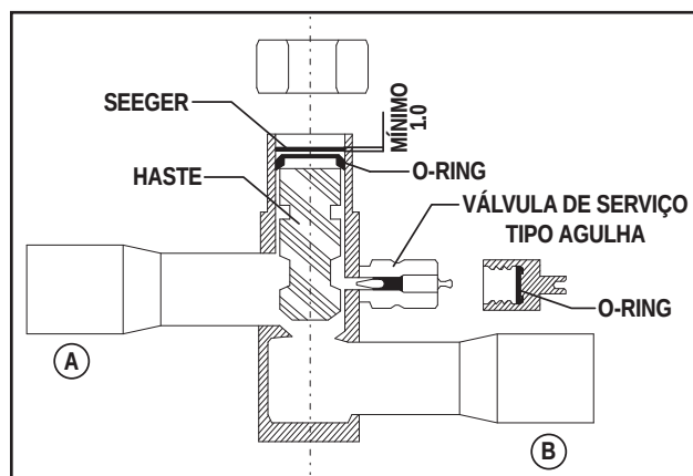
FIG. 28 - VÁLVULA DE SERVIÇO ABERTA
