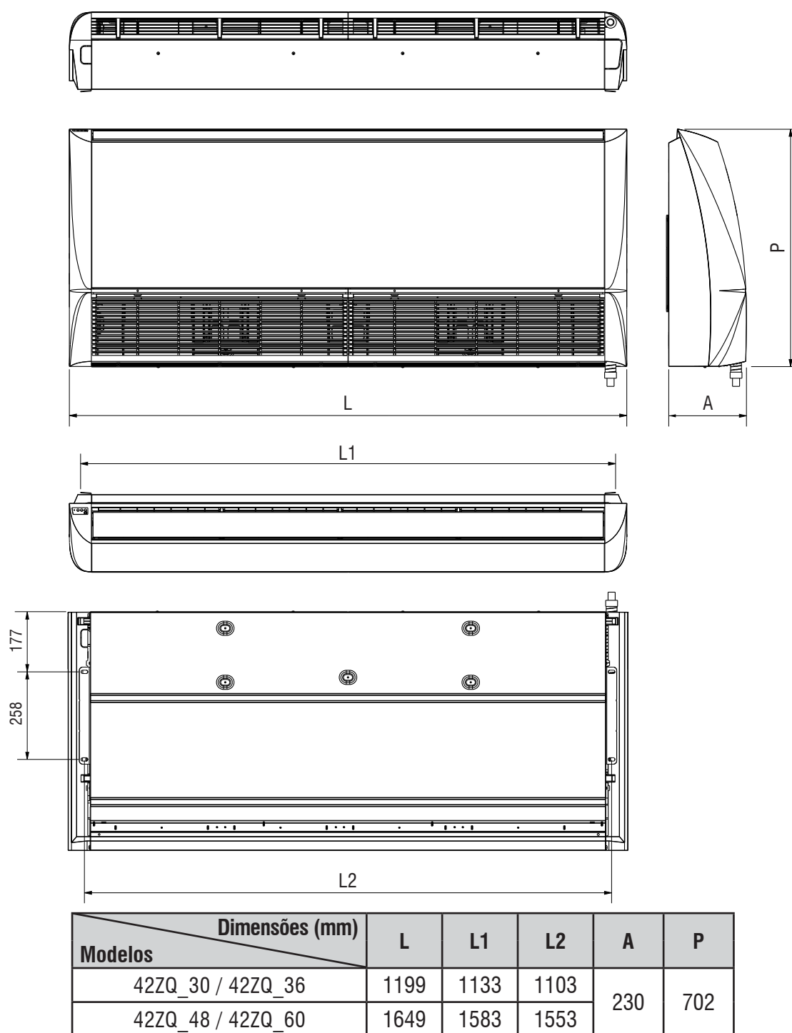
FIG. 14 - DIMENSIONAL UNIDADE EVAPORADORA
