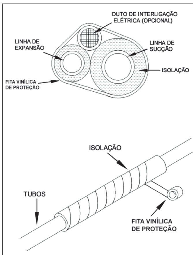
FIG. 39 - TUBULAÇÃO DE INTERLIGAÇÃO
