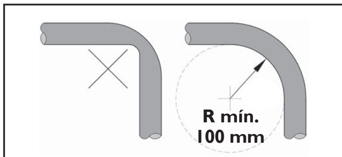
FIG. 38 - TUBULAÇÃO DE INTERLIGAÇÃO
