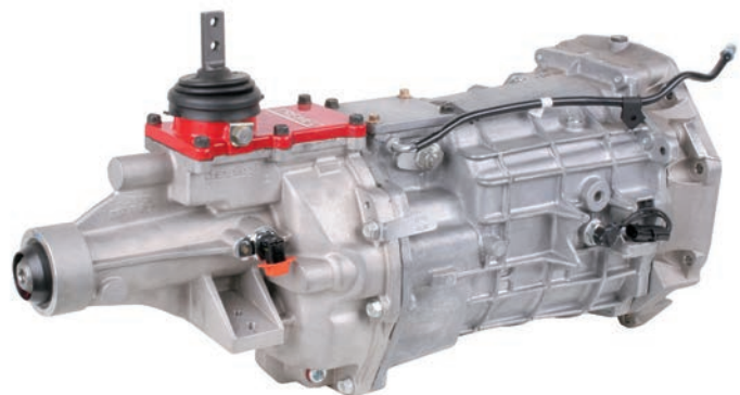
M-7003-M6295 shown
