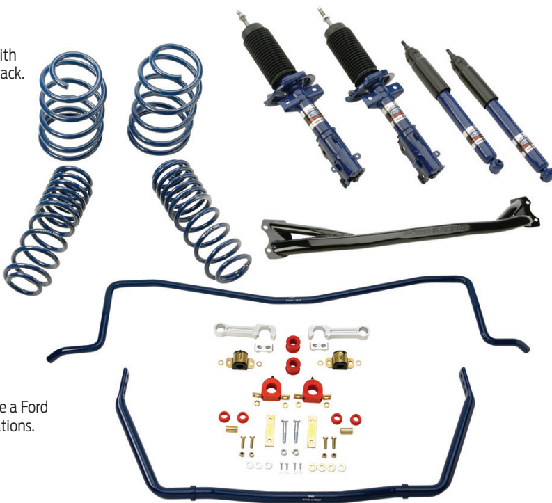
M-FR3-MSVTA shown
