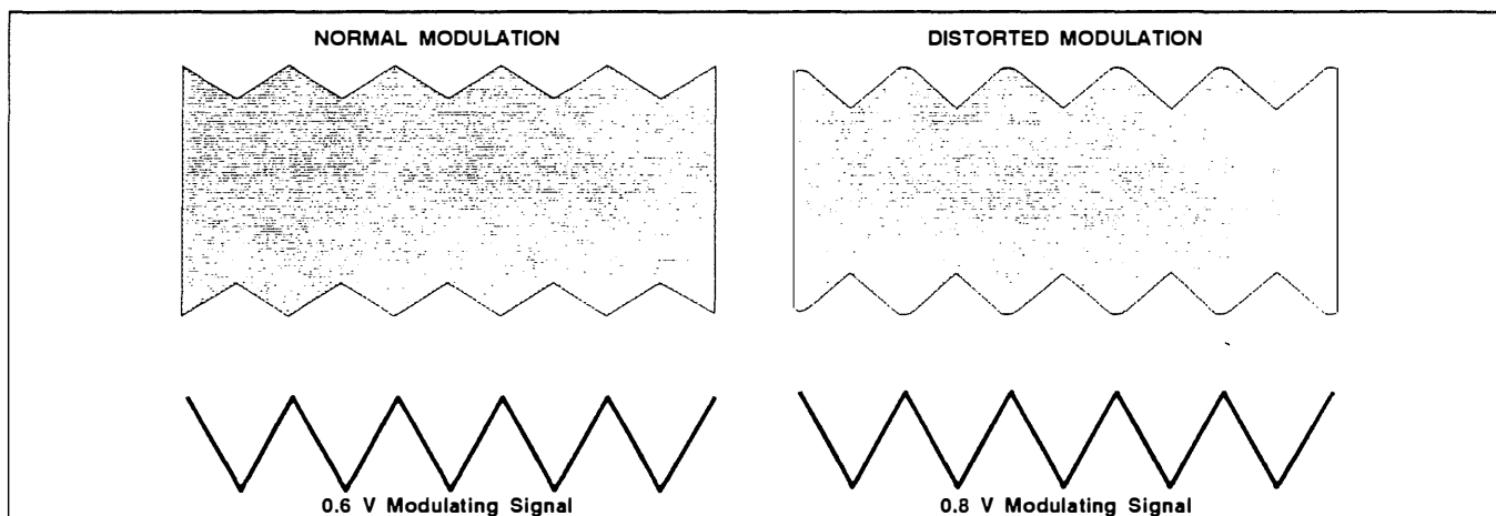
Fig. 2-7. AM Distortion.
