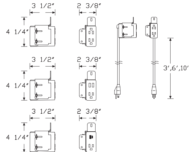
Grommet Mount
