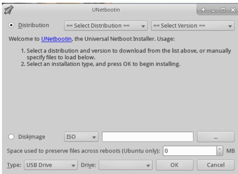
Figura 2-2: Unetbootin
