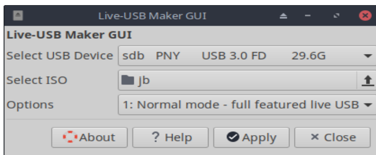
Figura 3-12: Construir LiveUSB
