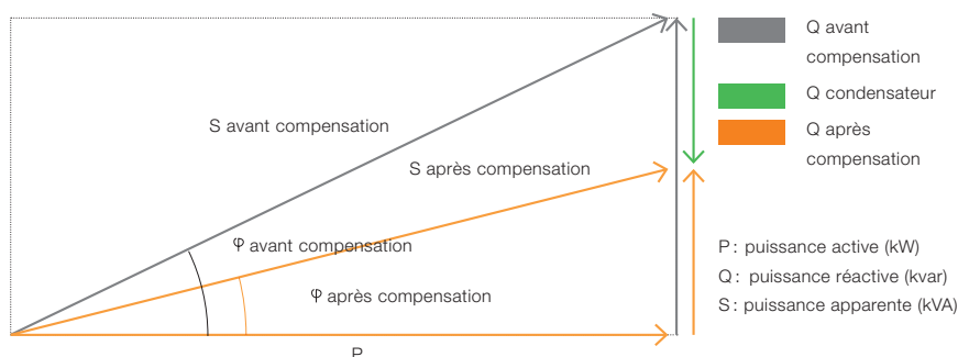
b Les condensateurs servent à compenser le déphasage provoqué par les moteurs électriques.
